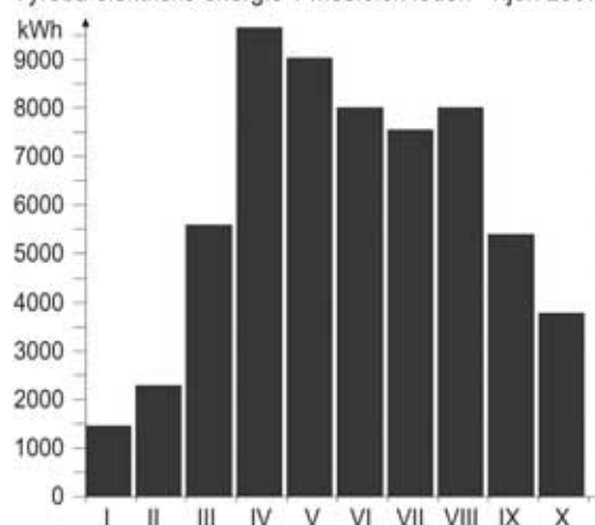
Výroba elektrické energie v měsících leden - říjen 2007
